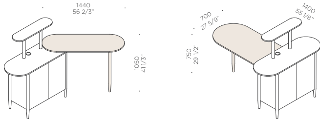
en_Table H. 1050 mm - 41 1/3" it_Tavolo H. 1050 mm - 41 1/3" fr_Table H. 1050 mm - 41 1/3" en_Table H. 750 mm - 29 1/2" it_Tavolo H. 750 mm - 29 1/2" fr_Table H. 750 mm - 29 1/2"
