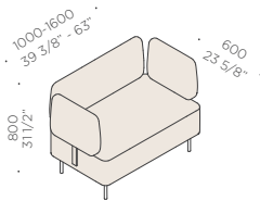
en_Sofa with armrests it_Divano con braccioli fr_Canapé avec accoudoirs
