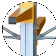
Les tubes sont boulonnés à l'oreille de part et d'autre de la colonne
