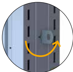
L'oreille est insérée à l'horizontale puis pivotée verticalement
