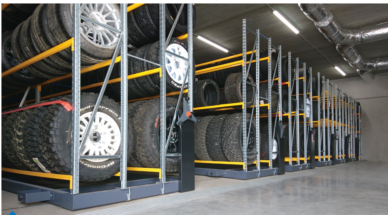
Stockage de pneumatiques sur rayonnage mi-lourd avec echelles ouvertes, butées, colonne gris anthracite.
