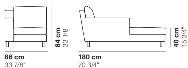
cod. 5115 / left small dormeuse
