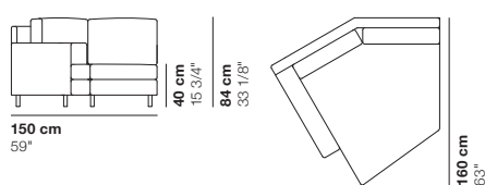
cod. 5117 / left big dormeuse
