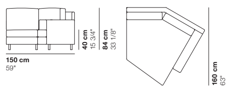
cod. 5116 / right big dormeuse
