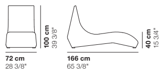
cod. 5705 / dormeuse
