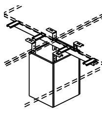
basamento per piani doppi double top base base pour plateau double base para sobre doble
